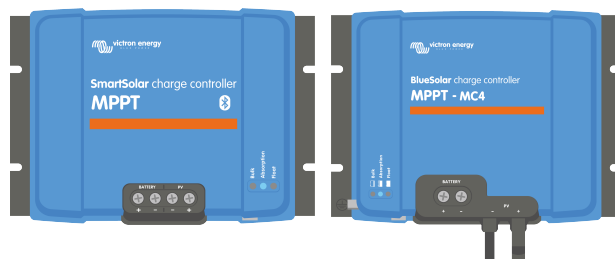
De gauche à droite : Exemple de chargeurs solaires avec des bornes à vis et des connexions PV MC4
